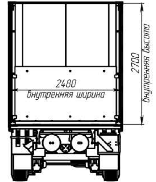
Б-Б (1 : 50)
